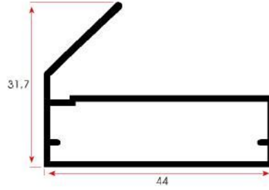
FSM 937 / 0,465 kg/m
