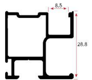
FSM 1017 0,470 kg/m
