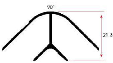
FSM 802 0,245 kg/m
