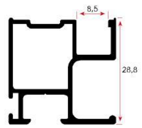
FSM 1017 0,470 kg/m
