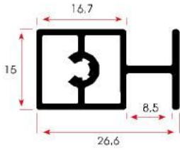
FSM 1018 0,341 kg/m
