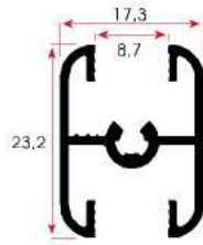
FSM 1035 0,272 kg/m
