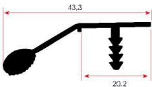
FSM 323 0,395 kg/m
