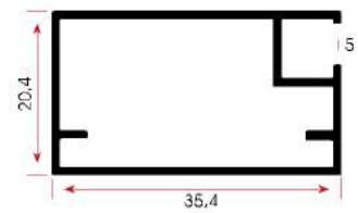
FSM 912 0,366 kg/m
