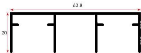
FSM 229 / 0,487 kg/m
