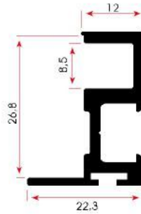
FSM 1016 0,465 kg/m
