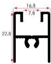
FSM 1026 0,265 kg/m
