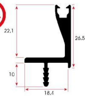
FSM 326 0,381 kg/m
