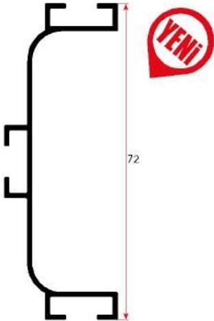
FSM 823 0,655 kg/m
