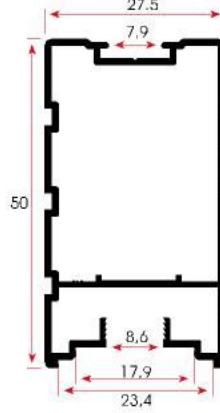
FSM 1021 0,550 kg/m
