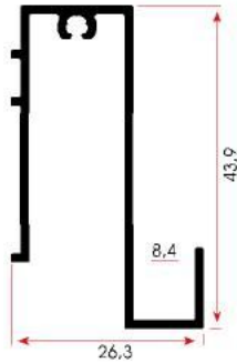
FSM 1020 0,410 kg/m
