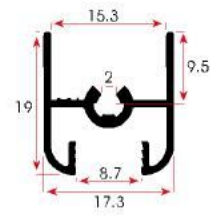
FSM 1036 0,204 kg/m
