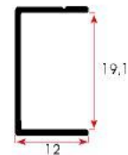
FSM 335 0,116 kg/m
