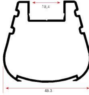
FSM 702 0,628 kg/m
