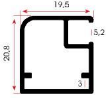
FSM 901 0,287 kg/m
