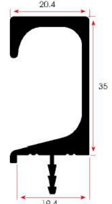
FSM 339 0,595 kg/m
