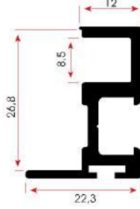
FSM 1016 0,465 kg/m
