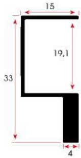
FSM 316 0,262 kg/m
