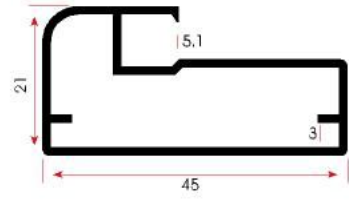
FSM 905 0,452 kg/m
