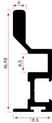
FSM 1015 0,670 kg/m
