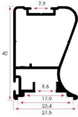
FSM 1022 0,515 kg/m
