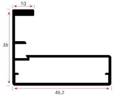
FSM 920 / 0,520 kg/m
