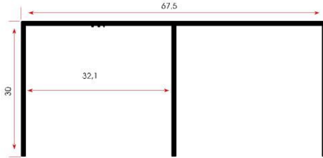
FSM 1011 0,457 kg/m
