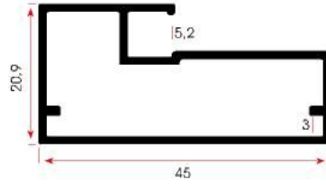
FSM 904 0,430 kg/m
