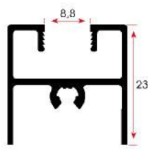
FSM 1013 0,312 kg/m
