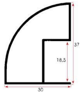
FSM 334 0,350 kg/m
