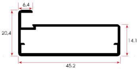
FSM 919 / 0,450 kg/m
