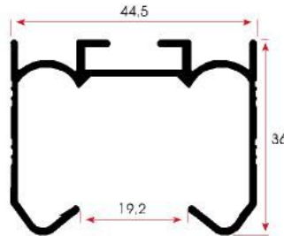
FSM 211 / 0,625 kg/m
