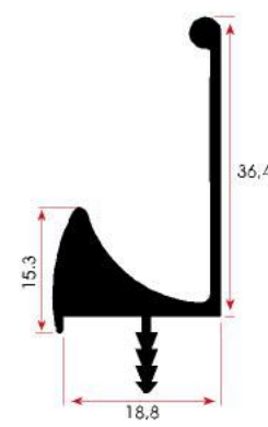
FSM 321 0,515 kg/m
