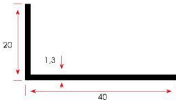
FSM 107 0,207 kg/m
