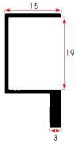
FSM 337 0,210 kg/m
