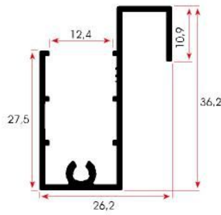
Alt-Üst Bağlantı
