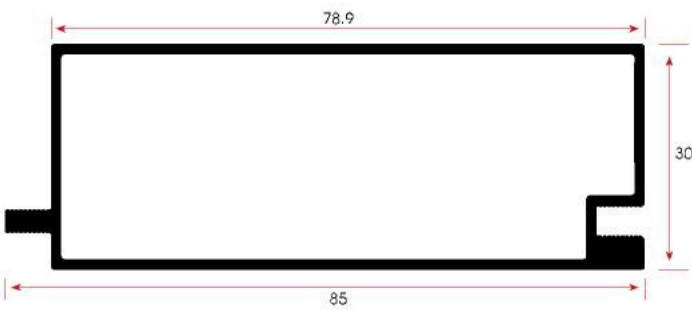
FSM 1503 0,937 kg/m
