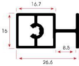
FSM 1018 0,341 kg/m
