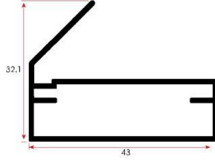
FSM 937 / 0,465 kg/m
