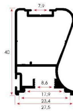
FSM 1022 0,515 kg/m
