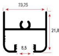
FSM 1004 0,265 kg/m
