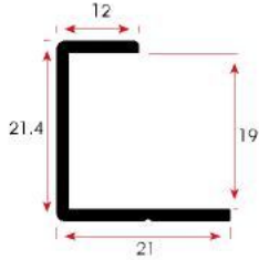
FSM 319 0,169 kg/m
