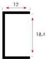
FSM 409 0,127 kg/m
