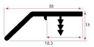
FSM 325 0,375 kg/m
