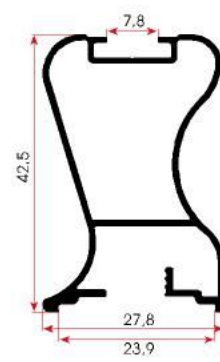
FSM 1041 0,450 kg/m
