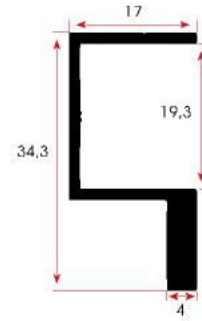
FSM 315 0,347 kg/m
