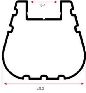
FSM 701 0,637 kg/m
