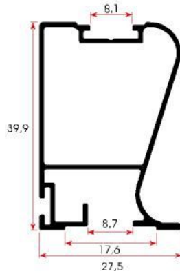
FSM 1027 0,500 kg/m
