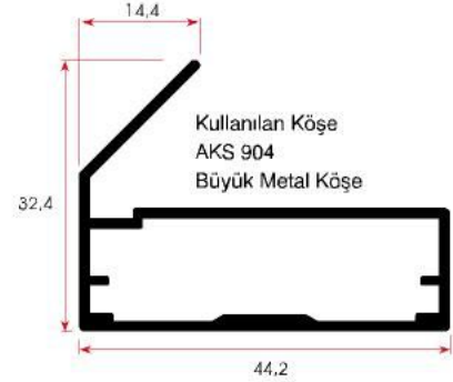
FSM 908 / 0,525 kg/m
