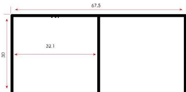
FSM 1011 0,457 kg/m
