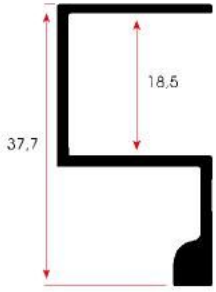
FSM 313 0,335 kg/m
