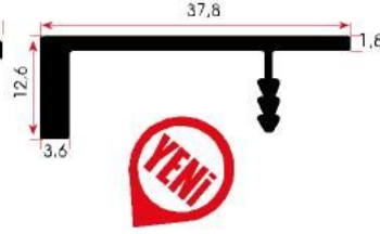
FSM 352 0,345 kg/m
