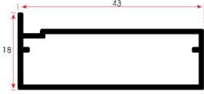
FSM 936 / 0,395 kg/m
