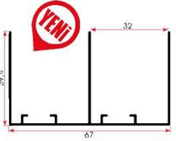
FSM 234 0,553 kg/m
