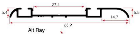
FSM 1031 0,254 kg/m
