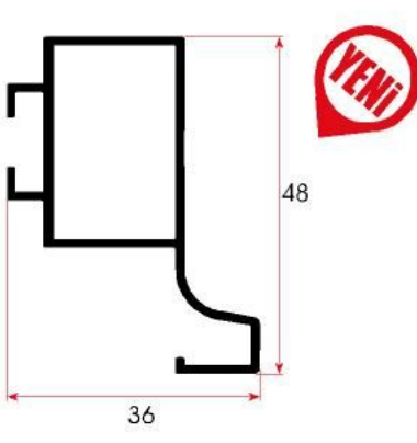
FSM 824 0,526 kg/m
