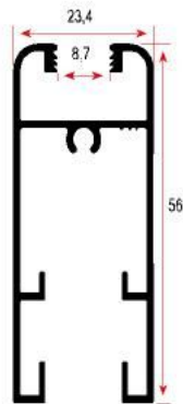
FSM 1021 0,550 kg/m
