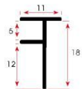
FSM 419 0,097 kg/m
