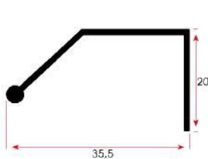
FSM 324 0,207 kg/m
