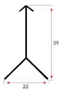
FSM 422 0,225 kg/m
