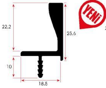
FSM 351 0,340 kg/m
