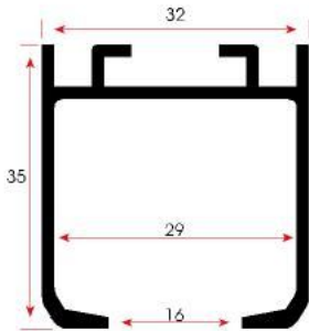
FSM 209 / 0,522 kg/m
