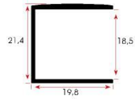
FSM 317 0,205 kg/m
