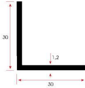
FSM 105 0,191 kg/m
