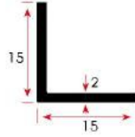
FSM 102 0,151 kg/m
