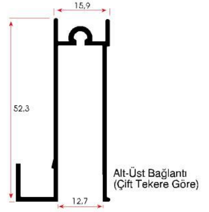
FSM 1033 0,510 kg/m
