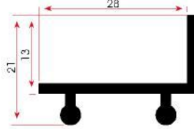
FSM 219 0,324 kg/m
