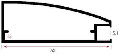
FSM 906 0,468 kg/m
