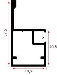
FSM 903 0,380 kg/m
