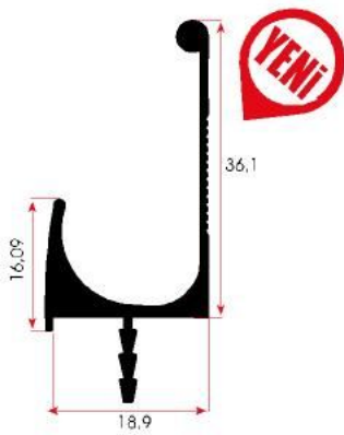
FSM 353 0,385 kg/m
