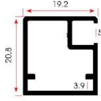
FSM 902 0,282 kg/m
