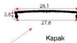
FSM 1032 0,087 kg/m
