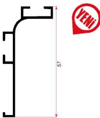
FSM 822 0,362 kg/m
