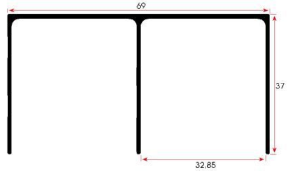
FSM 1025 0,550 kg/m
