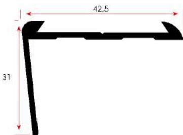
FSM 110 0,375 kg/m
