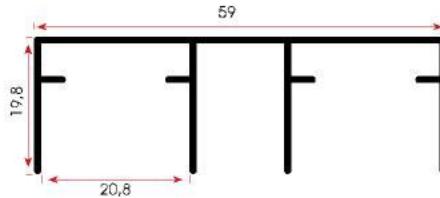
FSM 213 / 0,413 kg/m
