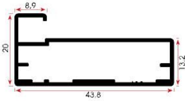
FSM 934 0,450 kg/m
