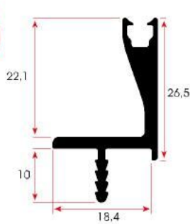
FSM 326 0,381 kg/m
