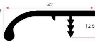
FSM 312 0,405 kg/m
