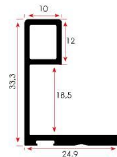
FSM 332 0,406 kg/m
