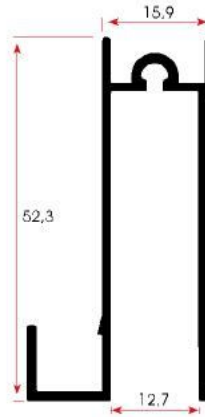
FSM 1033 0,510 kg/m
