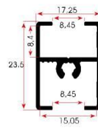
FSM 1028 0,265 kg/m
