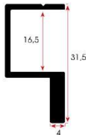
FSM 328 0,330 kg/m
