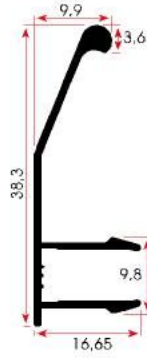
FSM 935 0,210 kg/m
