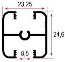
FSM 1003 0,325 kg/m
