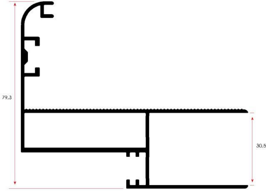
FSM 1501 1,021 kg/m
