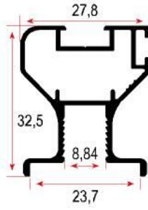
FSM 1002 0,400 kg/m
