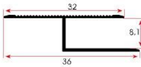
FSM 117 0,139 kg/m
