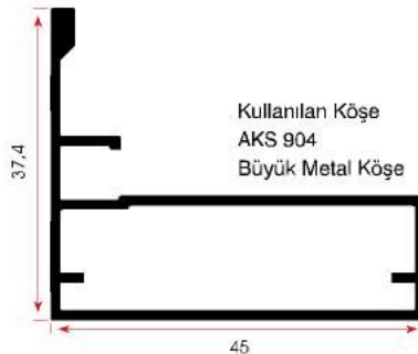
FSM 911 0,520 kg/m
