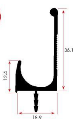
FSM 322 0,415 kg/m
