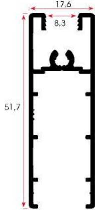
FSM 1008 0,253 kg/m
