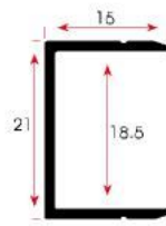
FSM 320 0,160 kg/m
