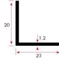
FSM 103 0,128 kg/m
