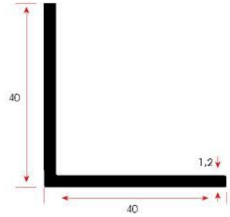
FSM 106 0,256 kg/m
