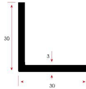
FSM 108 0,463 kg/m
