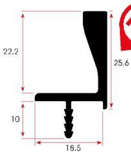
FSM 351 0,340 kg/m
