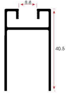
FSM 1014 0,397 kg/m
