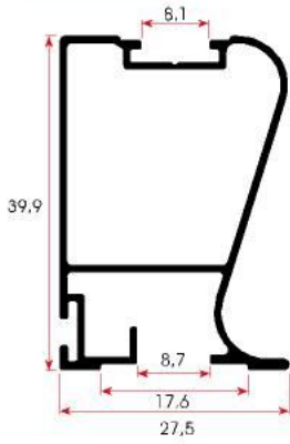
FSM 1034 0,425 kg/m
