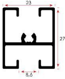
FSM 1012 0,376 kg/m
